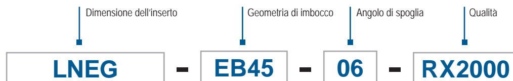
Inseri LNEG per testine Xfix HF86 e HF86B
