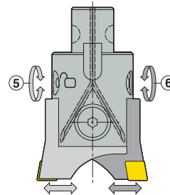
Regolazione indipendente
