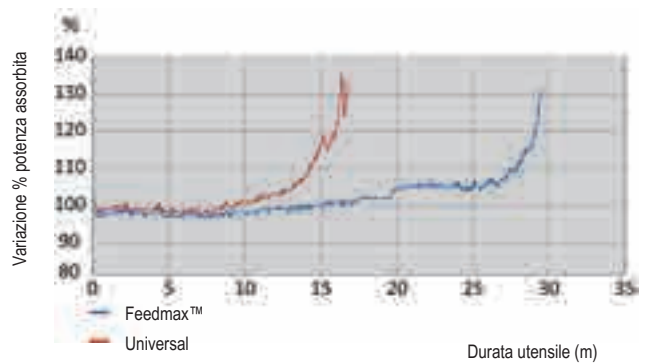
Durata con parametri di taglio alti
