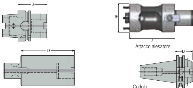
Prolunga
