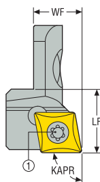
1 = Vite di bloccaggio inserto
