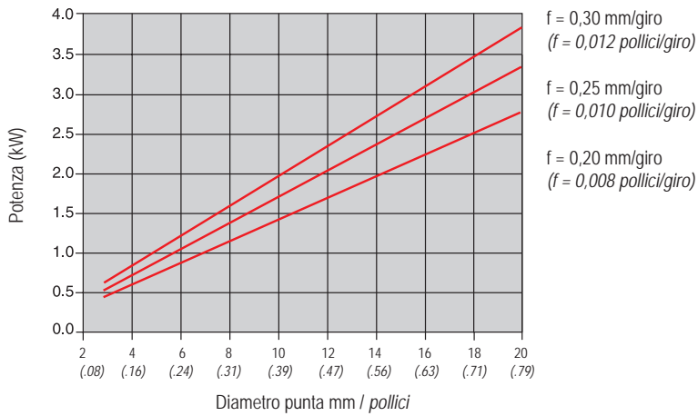
Potenza assorbita
