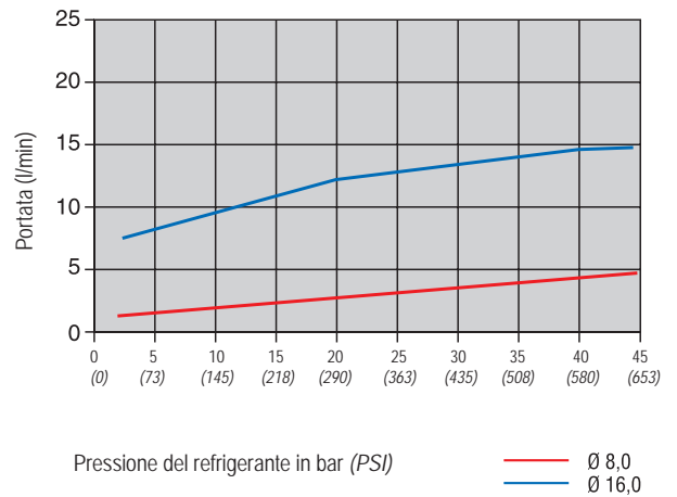
Portata refrigerante a diverse pressioni
