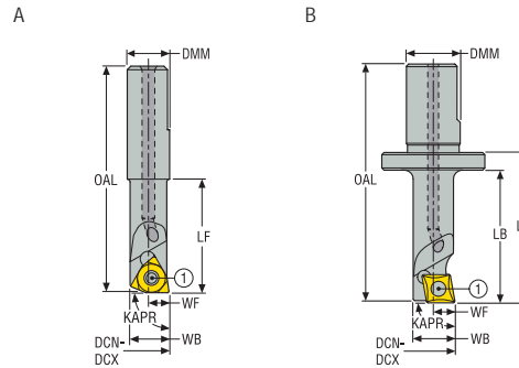
1 = Vite di bloccaggio inserto
