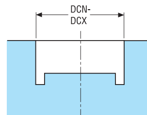
Utensile per scanalatura -verso foro-
