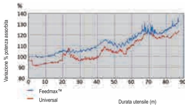
Durata con parametri di taglio bassi
