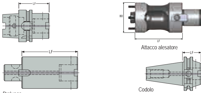
Prolunga
